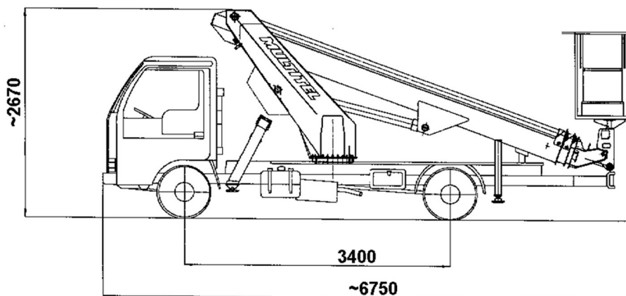
NISSAN CABSTAR 110.35 - 3400 mm
