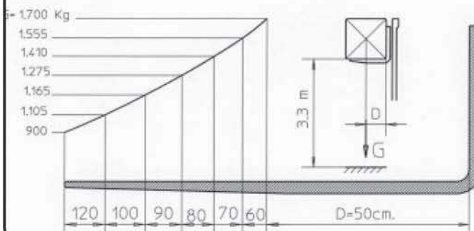
CUADRO DE CARGAS LOAD CHART TABLEAU DE CHARGEMENTS
